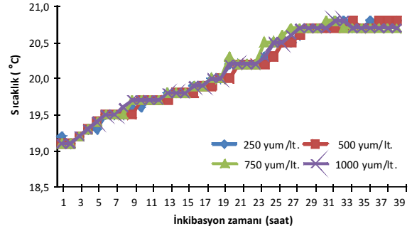
Şekil 1. Denemeler süresince inkibatörlerde meydana gelen sıcaklık değişimi.
