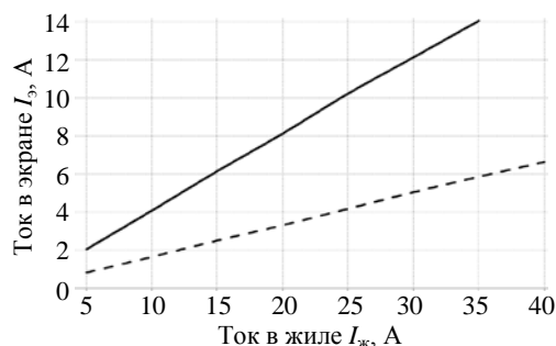
Рис. 5. Зависимость индуцируемого тока в экране от тока в жиле: — s = 32 \text{ мм}^2 ; - - - 16 \text{ мм}^2
