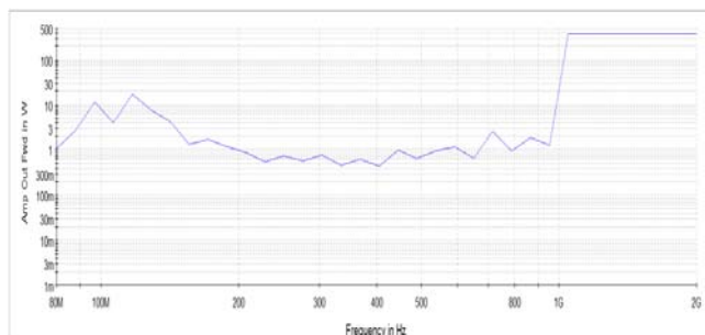
Fig. 6. Amp Out Fwd – test 1.
