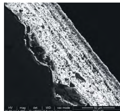
fig. 1. Costra criptocristalina de schuetteita (clara) mostrando bandeo rítmico, con abundantes granos de cuarzo, illita y caolinita (granos más oscuros), que se interpretan como restitidos del substrato cuarcítico (más oscuro, izquierda). Escombrera de El Entredicho. SEM, modo BSE.
