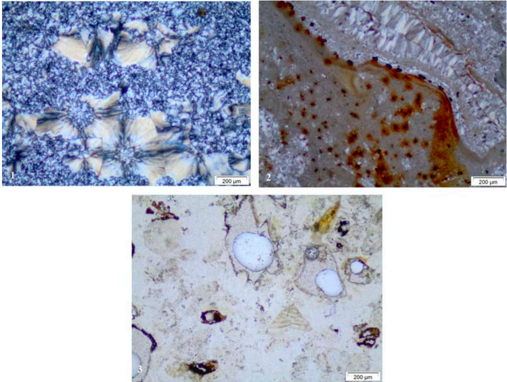
Fig. 5. Láminas delgadas de tres muestras de la Dolina de l'Esquerda de les Alzines. 1) LP 335: sílex continental/evaporítico, matriz de microcuarzo y esferulitas rellenoando cavidades. 2) LP 400: raspador de sílex calcedónico, con bandas de matriz micrítica atravesadas por bandas calcedónicas. 3) LP 851: sílex moteado, matriz micrítica con Pattellina .
