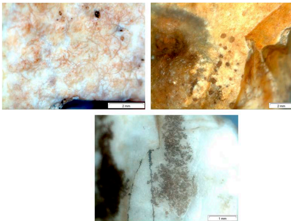
Fig. 2. 1) Marcas semicirculares de grosor fino. 2) Pseudomorfos romboidales de calcita/dolomita. 3) Dendritas de manganeso.
