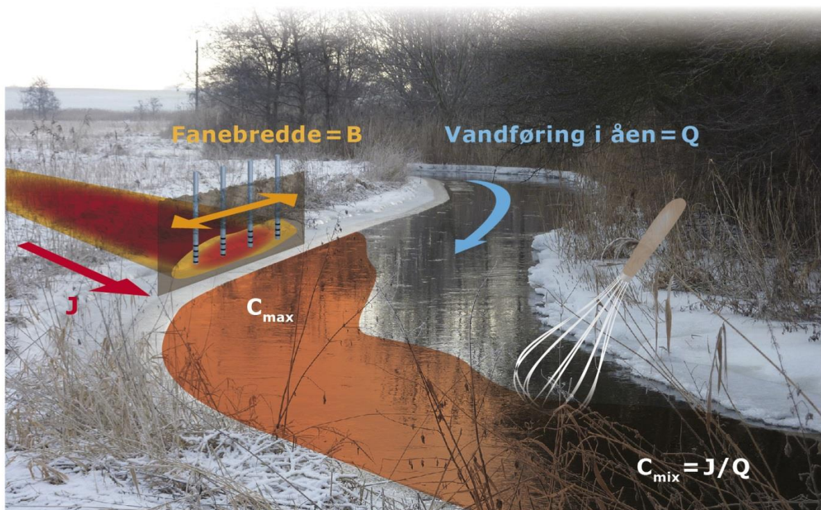
Figur 1: Konceptuel model for udsivning af en punktkildeforurening til et vandløb. Koncentrationen, C_{mix} , i vandløbet kan under antagelse af fuld opblanding beregnes som C_{mix} = J/Q , hvor J er forureningsfluxen og Q er vandføringen i vandløbet
