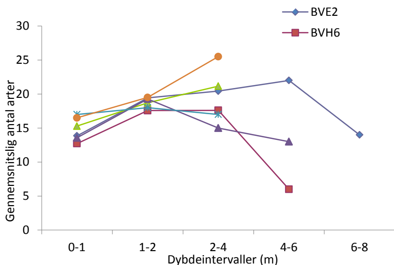
Figur 5. Antal arter fordelt på dybdeintervaller på de seks transekter i Natura 2000 området (N56) ved Horsens i perioden 2007-2015 (Data fra Naturstyrelsen Kronjylland).
