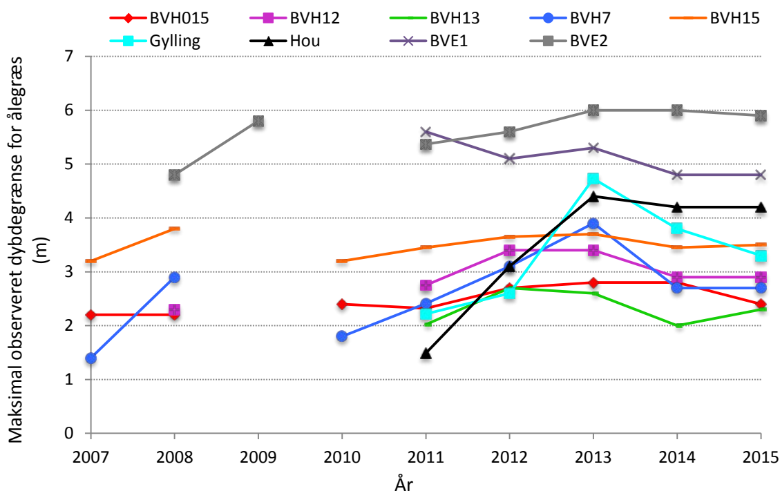
Figur 3. Den maksimale dybdeudbredelse for ålegræs på transekter i og umiddelbart nærhed af Natura 2000 området ved Horsens i perioden 2007-2015 (Naturstyrelsen Kronjylland, 2015). Transekt BVH7 og BVH015 ligger begge lige udenfor Natura 2000, mens de resterende 7 transekter ligger indenfor Natura 2000 området (N56).
