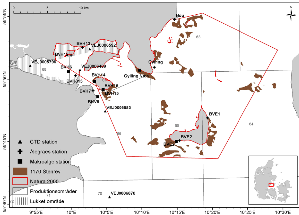
Figur 1. Natura 2000 område N56 ved Horsens. De kortlagte stenrev, lukkede område og muslingeproduktionsområder er vist. Derudover er placeringen af ålegræs- og makroalgetransekter (hhv. + og ■) samt CTD-stationer (▲) angivet. Det er kun stationer og transekter indenfor eller i umiddelbar nærhed af Natura 2000 området (N52), som er blevet monitoreret indenfor den seneste årrække, der er angivet.
