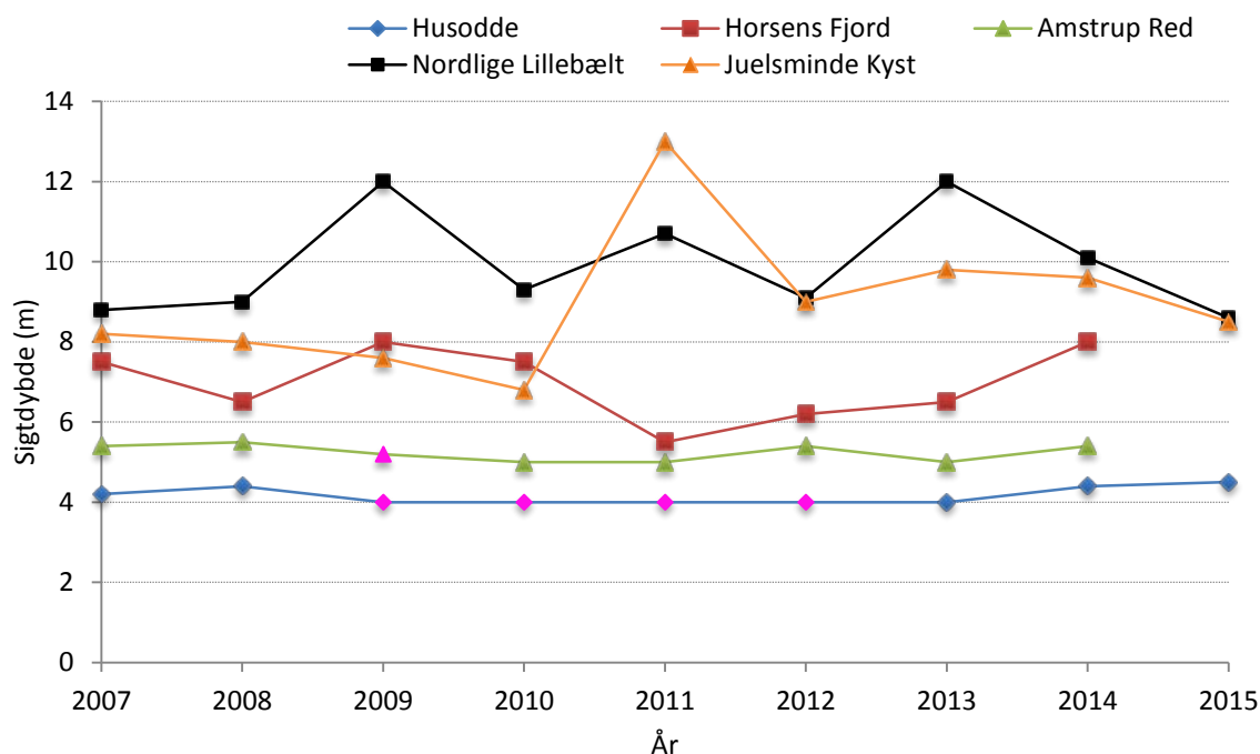
Figur 4. Den gennemsnitlige sigtdybde i eller tæt ved Natura 2000 området (N56) ved Horsens i perioden 2007-2015. Den gennemsnitlige sigtdybde inkluderer kun data fra ålegræssets vækstperiode (marts-oktober). Bemærk, at et pink datapunkt angiver sigtdybde til bunden for det pågældende år.
