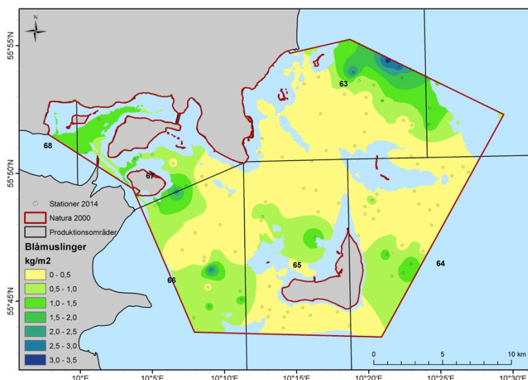
Figur 6. Udbredelseskort, der viser fordelingen og tætheden af blåmuslinger på vanddybder større end 3 m og mindre end 15 m i Natura 2000 området N56 ved Horsens i juni 2014.
