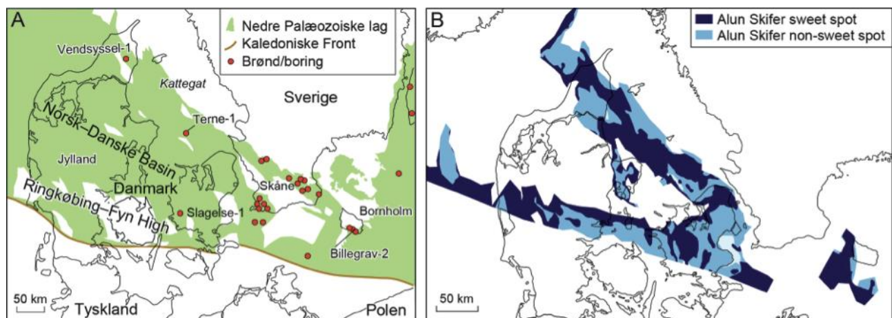
Figur 4. A) Geologisk kort der viser udbredelsen af palæozoiske bjergarter. Kortet viser også borer, der gennemborer Alun Skiferen. B) Prospektivt område i Danmark for skifergas med angivelse af bruttoudbredelsen af "sweetspots" og "non-sweetspots" (defineret i tekst, se også figur 6). Kort efter Schovsbo et al. (2011, 2014).
