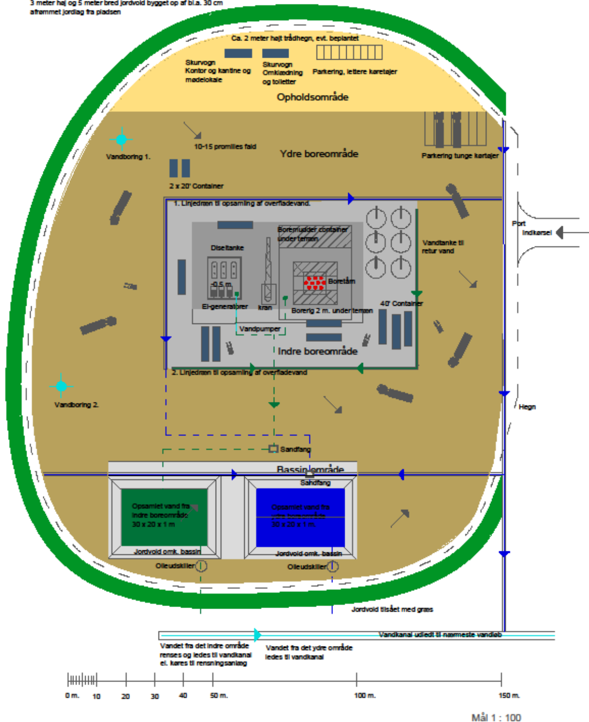
Figur 22: Illustration af muligt design og indretning af en skifergas boreplads i Danmark efter "Best Management Practices" imens der boret horisontalt.
