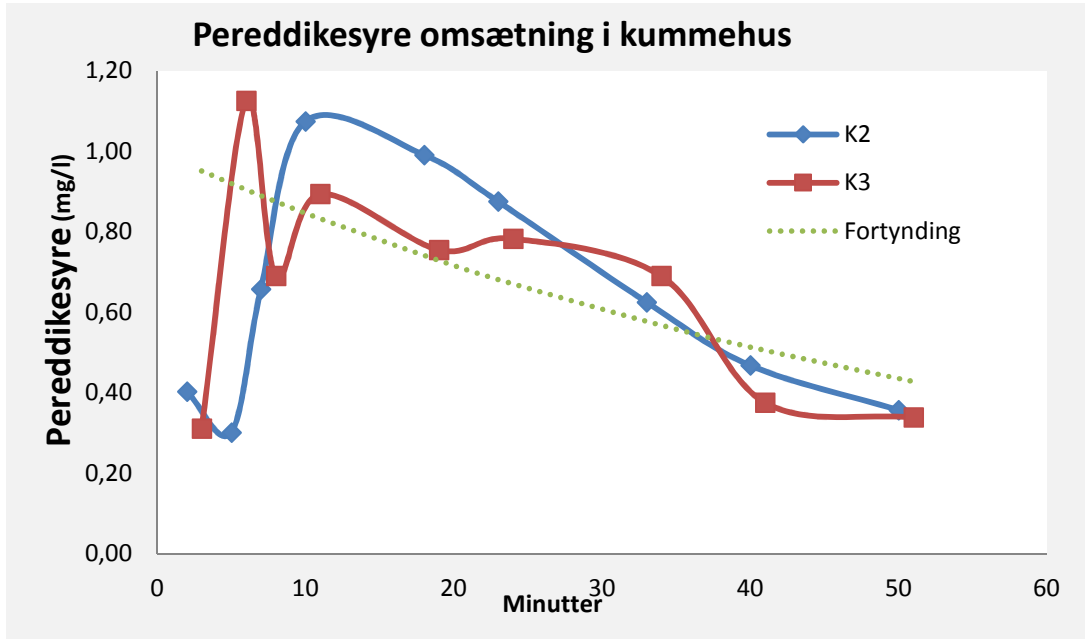
Fig. 5.3.9. Målte koncentrationer af pereddikesyre i kumme 2 og 3 i forbindelse med vanlig vandbehandling. Den stiplede linje angiver teoretisk koncentrationsforløb (startkoncentration = 1 mg/l, ingen omsætning; fortynding = 15 l/min).
