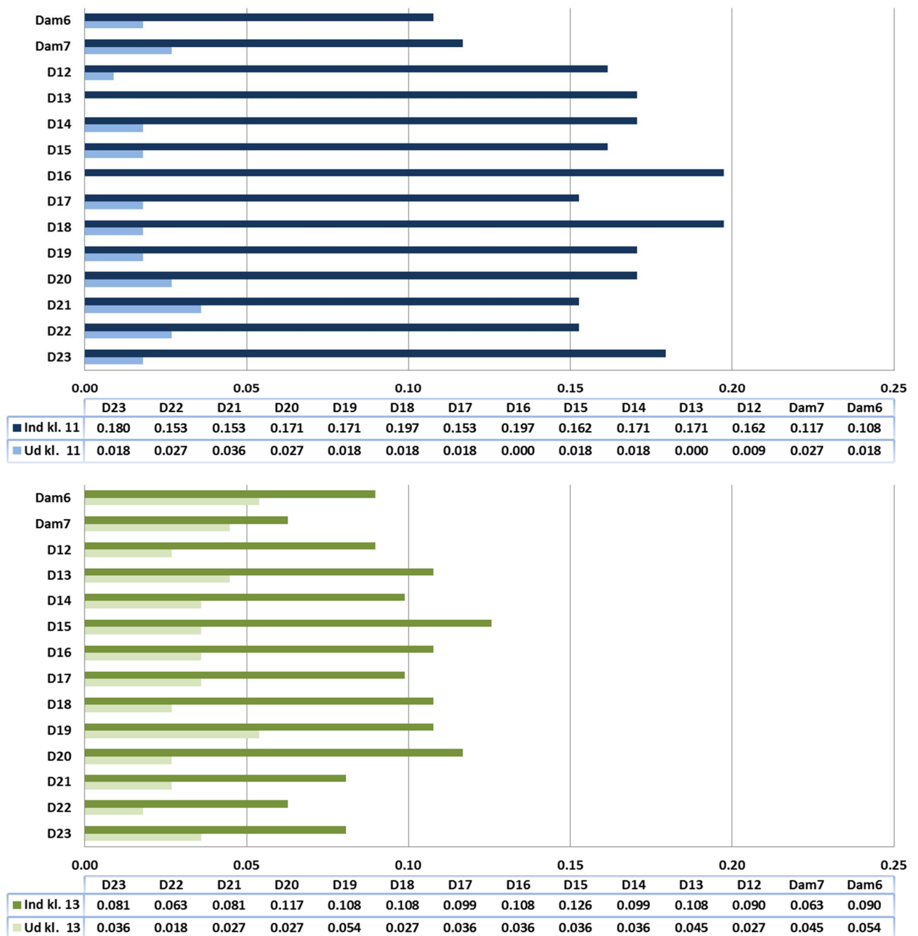
Figur 5.3.3. Måling af pereddikesyre på Kidmosebæk Dambrug den 31.maj 2013, formiddag (øverst) og eftermiddag (nederst). Det bemærkes at dam 6 og 7 ligger længst nedstrøms i forhold til doseringsstedet.
