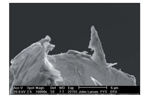
Scanning elektronmikroskopibilleder af en Pt/Ir probespids som dem vi bruger i vores scanning tunnel mikroskop. Nederst ses spidsen af proben med meget høj forstørrelse, bemærk hvor uregelmæssig probespidsen er.
