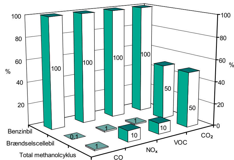
Figur 5. Emissioner fra en bil med methanoldrevet brændselle sammenlignet med en benzindrevet bil, hvor emissionerne er sat til 100%. Med "total methanolcyklus" menes samlede emissioner for hele processen fra fremstilling over distribution og forbrug af methanol. Det ses, at emissioner af carbonmonoxid (CO), nitrose gasser ( \text{NO}_x ) og flygtige organiske forbindelser (VOC, uforbrændt brændsel) er meget lavere for brændsellebilen. \text{CO}_2 -emissioner kan ikke undgås, da det er restproduktet for brændslet, men tallet er halveret p.g.a. brændsellellens større effektivitet og dermed mindre brændstofforbrug (Emons et al. J. Power Sources, 71, 288, 1998).
