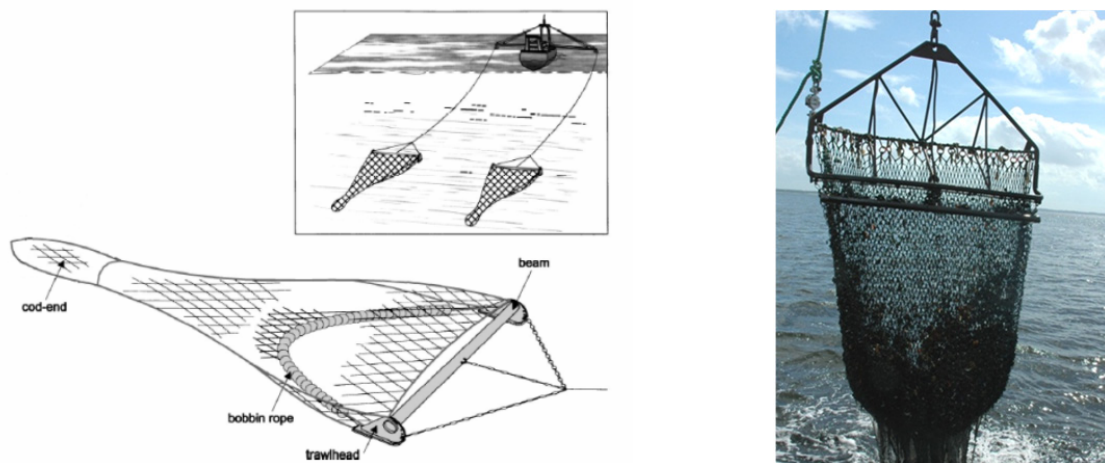
Figur 4.3.1. Bomtrawler til fiskeri efter hesterejer (til venstre), samt blåmuslingskraber (til højre). Se FAO(2014).
