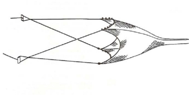
Figur 4.3.6. Pelagisk trawltype til bundnært fiskeri efter tobis, sild og brisling. Se FAO(2014).
