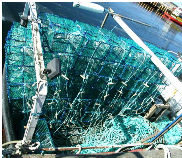
Fig. 4. Eidern Valborg klar til afgang med 5 lænker (125 tejner) rigget og klar til sætning. Færdsel på dækket undgås, så linerne ikke bliver viklet sammen. Af billedet ses vigtigheden af, at tjavsernes længder er afstemt efter bådens størrelse.
