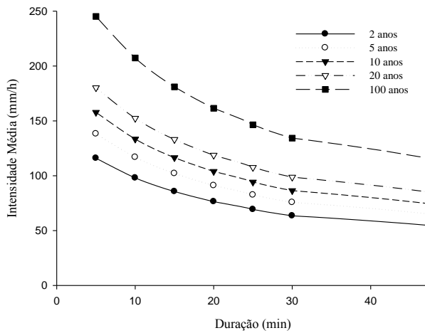
Figura 4. Curva IDF de Jaru (a) e de Machadinho do Oeste (b)
