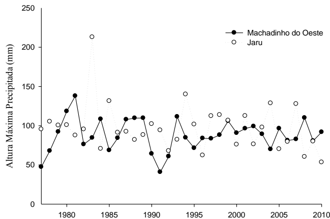
Figura 3. Série histórica da precipitação máxima de “um dia” por ano, para o município de Jaru e Machadinho d’Oeste
