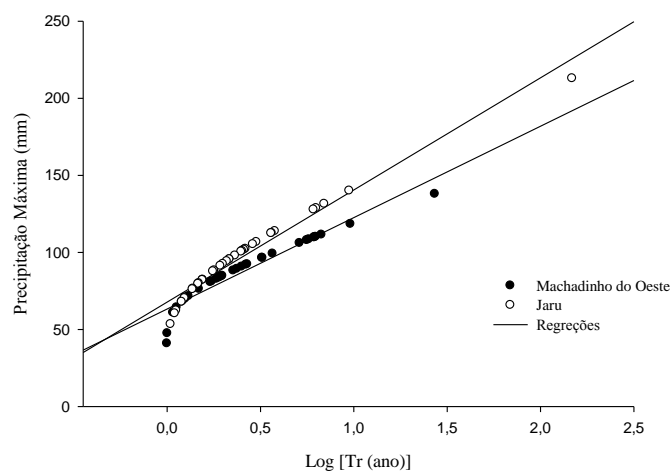
Figura 3. Retas de ajuste dos dados de precipitação máxima em relação ao período de retorno, para os municípios de Jarú e Machadinho d'Oeste
