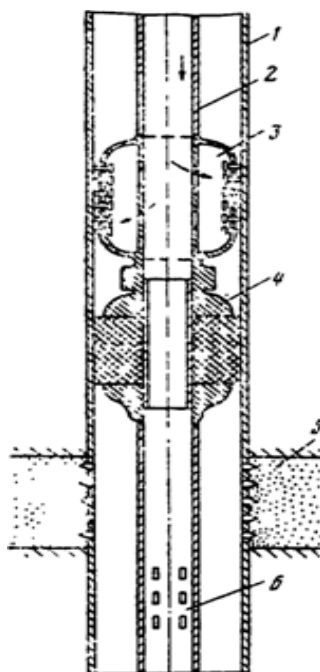
Рисунок 1.9 – Подземное оборудование для ГРП [7]
