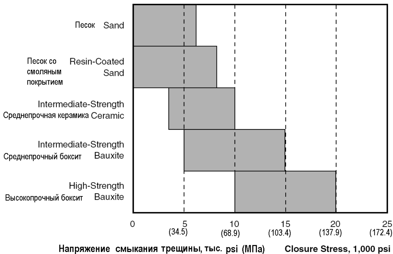
Рисунок 1.8 – Принцип выбора типа проппанта [4]
