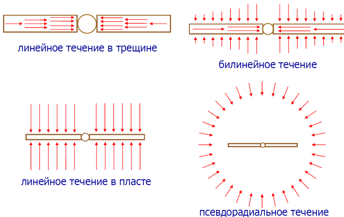
Рисунок 1.10 – Структуры потоков в пласте при ГРП [5]
