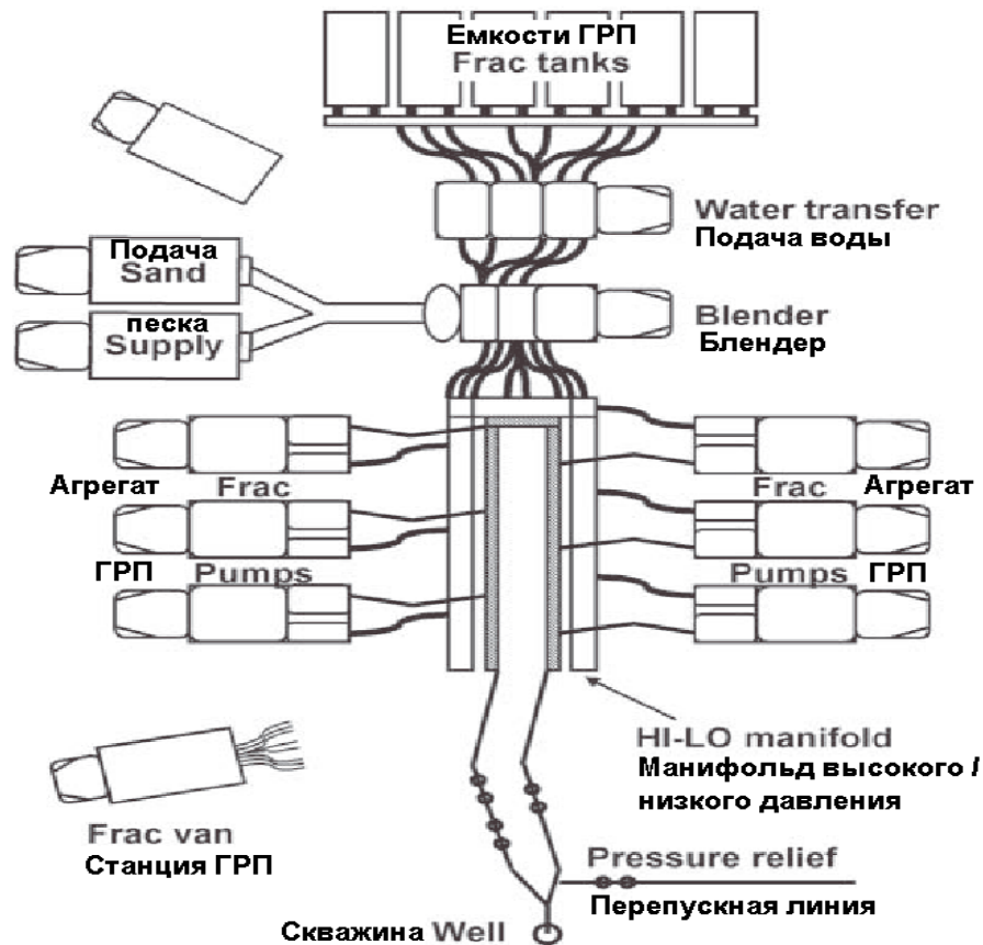
Рисунок 1.7 – Расположение оборудования ГРП [4]
