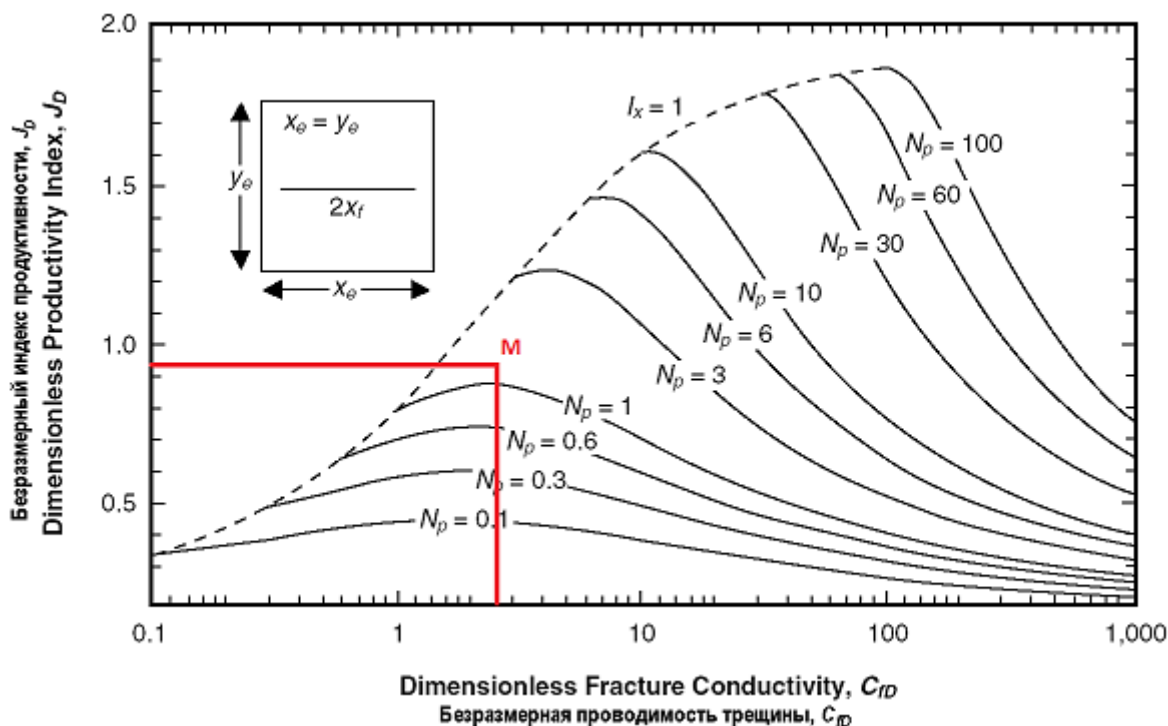
Рисунок 1.6 – Нахождение соответствующей точки М на графике [4]
