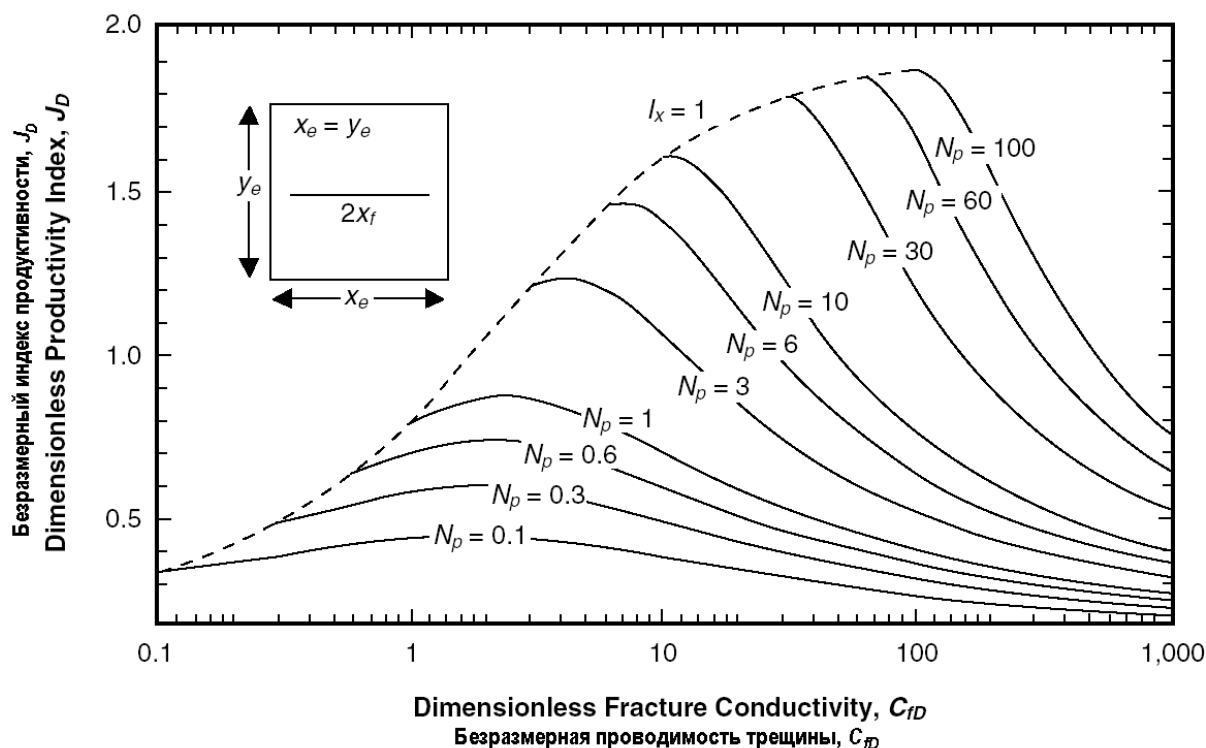
Рисунок 1.5 – Зависимость безразмерного индекса продуктивности от безразмерной проводимости трещины с постоянным количеством пропантанта[4]
