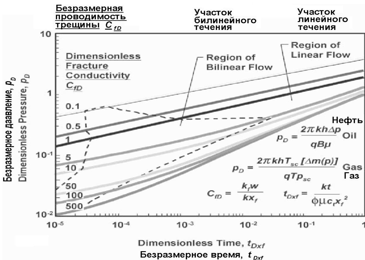
Рисунок 1.11 – Билогарифмический диагностический график для вертикальной скважины с ГРП [4]
