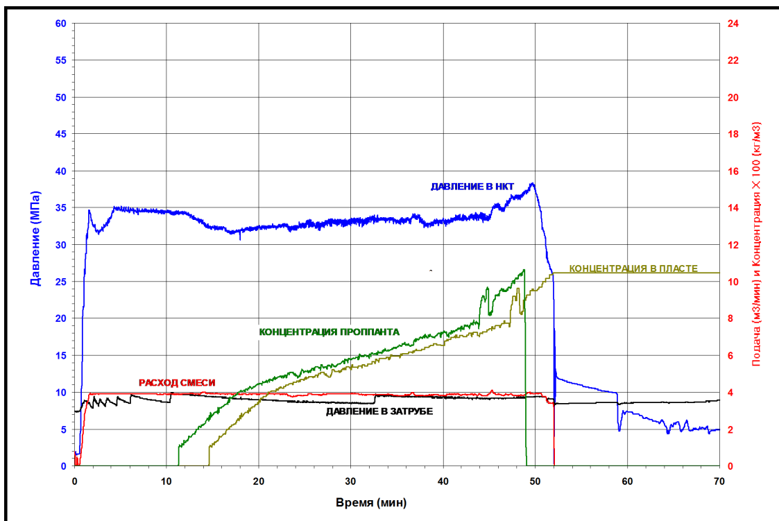
Рисунок 1.3 – Параметры на устье при ГРП [5]
