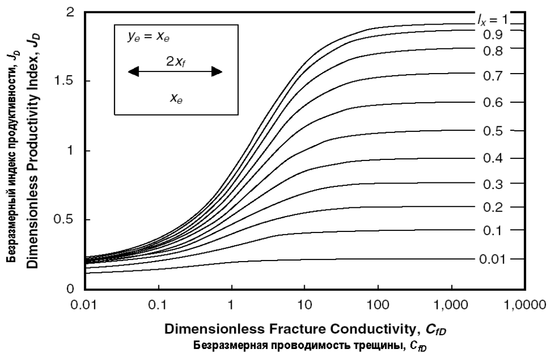
Рисунок 1.4 – Зависимость безразмерного индекса продуктивности от безразмерного проводимости трещины с различной степенью проникновения[4]
