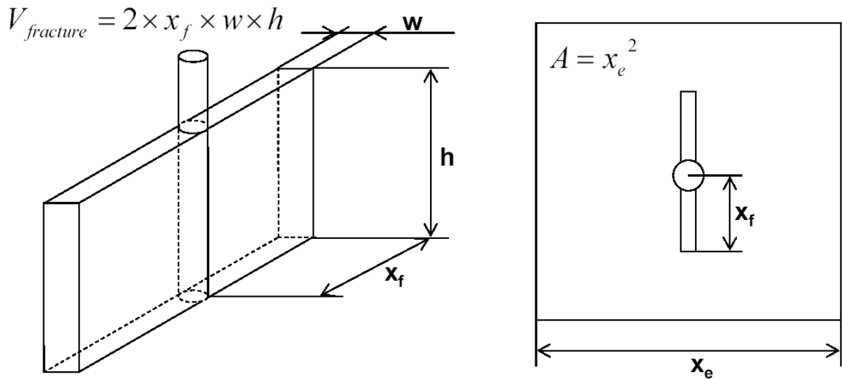
Рисунок 1.2 – Геометрия трещины ГРП [4]
