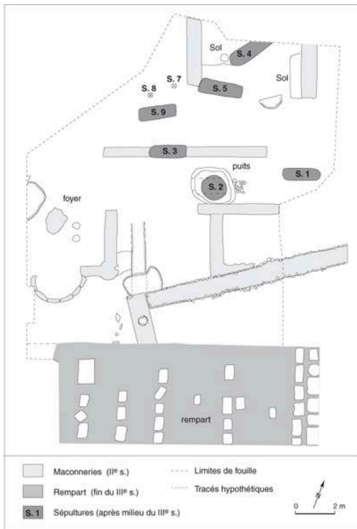
Fig. n°2 : Plan général des structures
