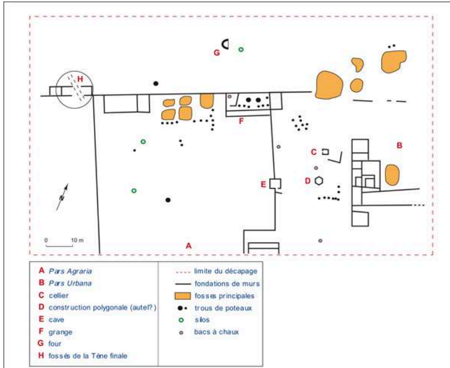
Fig. n°1 : Plan général du site
