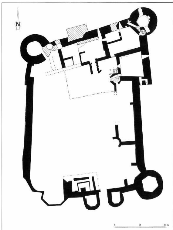
Fig. 1 – Plan du château (fouille 1998)
