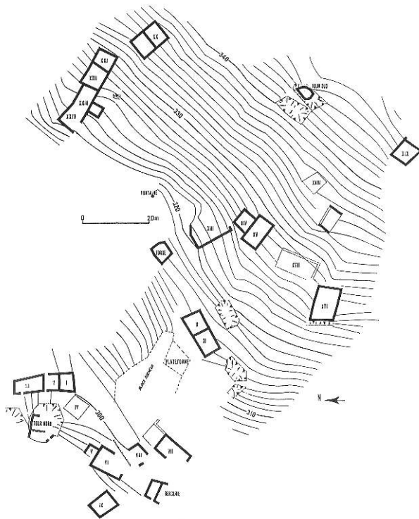
Fig. 1 – Plan d'ensemble du village de l'Ortolo
