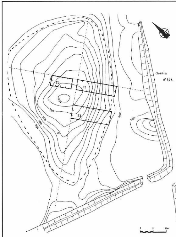
Fig. 1 – Relevé topographique du tertre et position des sondages S1, S2 et S3
