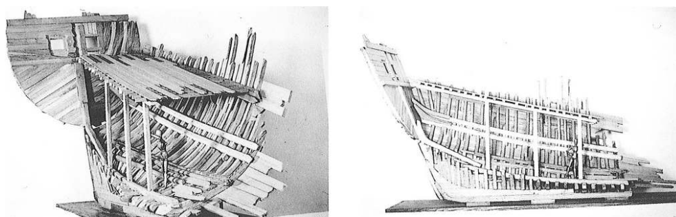
Fig. 1 – Maquette de la partie arrière du navire Calvi 1
