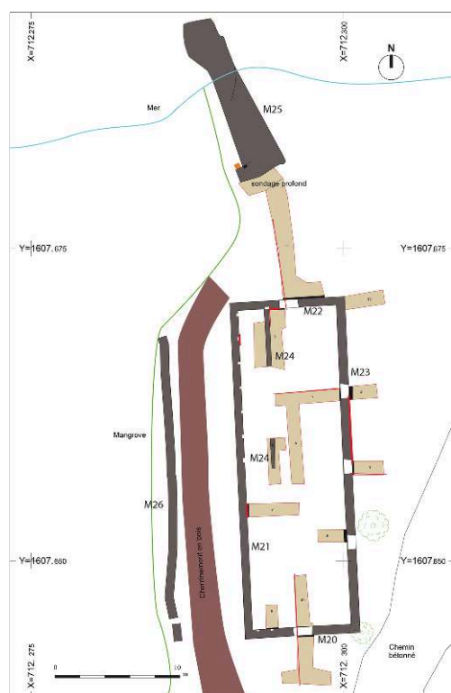
Fig. 1 – Plan général
