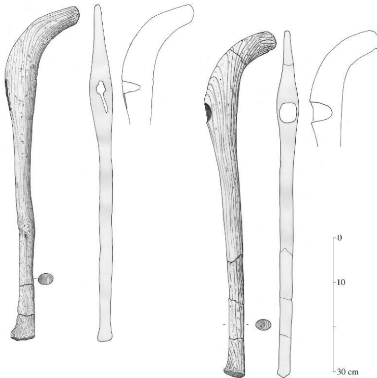
Fig. 2 – Clairvaux XIV : manches monoxyles de hache à tête recourbée en crosse
