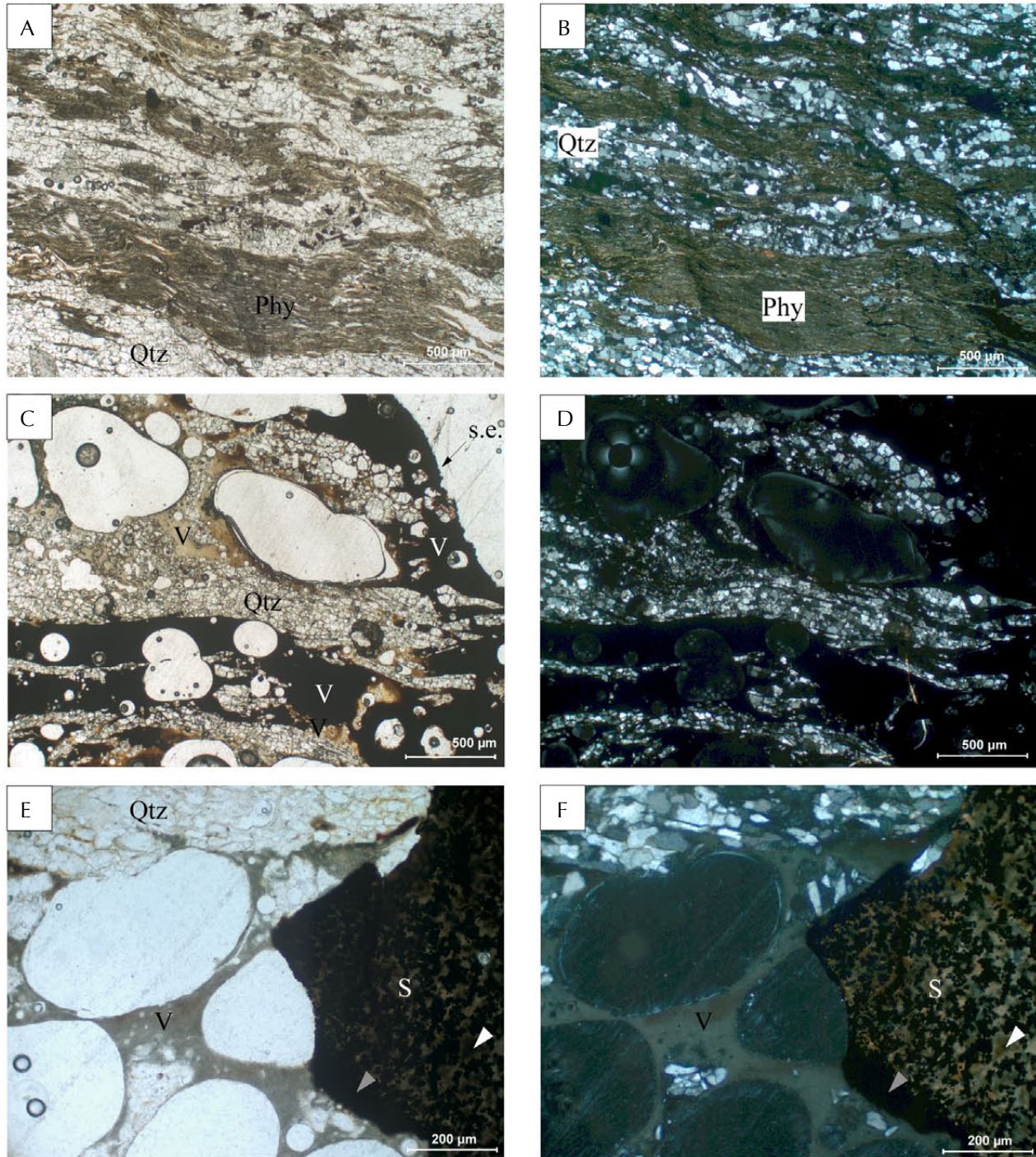
Fig. 11. Vues d'une lame mince du fragment de roche en microscopie optique. A (LPNA) et B (LPA) : zone non vitrifiée de la roche montrant l'alternance de lits de quartzite et de lits de phyllosilicates; C (LPNA) et D (LPA) : portion de la roche partiellement vitrifiée et scorie constituée principalement de verre opaque; E (LPNA) et F (LPA) : zoom sur la zone de soudure entre la scorie et la roche vitrifiée. Flèche blanche = verre + olivine dendritique; flèche grise: magnétite + verre (photos C2RMF/Y. Coquiot).
