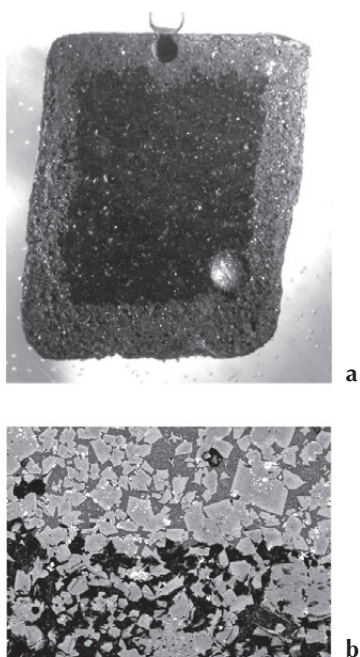
Fig. 9. a) Vue en coupe sous loupe binoculaire de la scorie 66033-2 montrant la corrosion affectant tout le pourtour de la scorie sur une profondeur pouvant atteindre 2 mm. b) Micrographie électronique en électrons retrodiffusés montrant un détail de la couche corrodée (en bas de l'image), qui révèle que seule la fayalite (en gris) a été épargnée (photos C2RMF/D. Bourgarit).
