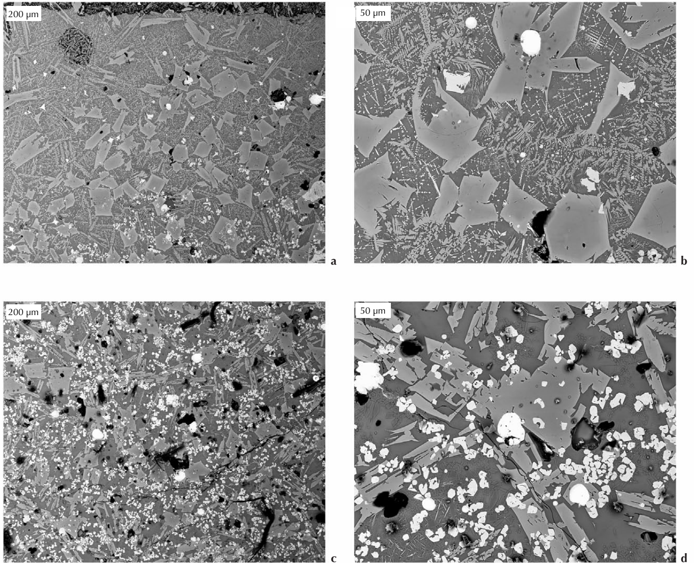
Fig. 10. Micrographies électroniques en électrons retroréfléchés montrant les trois phases cristallines principales dans les scories, à savoir la fayalite (en gris), la magnétite (en gris clair) et le cuivre métallique ou sous forme de sulfure (en blanc). Les morphologies des deux premières phases évoluent suivant leur localisation dans la scorie : a) zone sous la surface supérieure, b) détail de l'image précédente, c) microstructure typique dans le reste de la scorie, d) détail de l'image précédente montrant des cristaux de clinopyroxènes type hedenbergite (en gris foncé).
