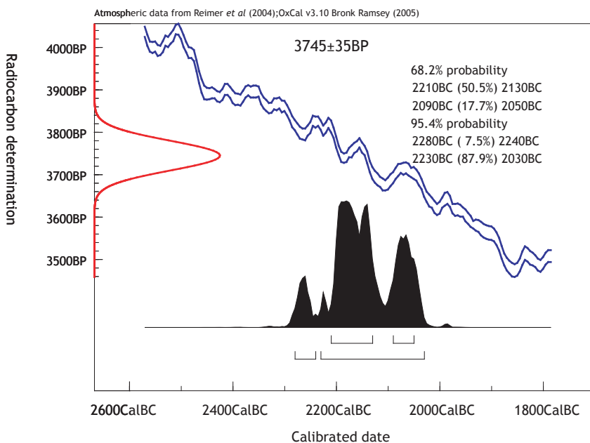
Fig. 5. Datation de l'Us 1008 du sondage 1 du vallon du Longet et compilation des principales datations publiées pour les sites miniers et métallurgiques du secteur de Saint-Véran (Hautes-Alpes) (DAO L. Carozza/A. Burens).
