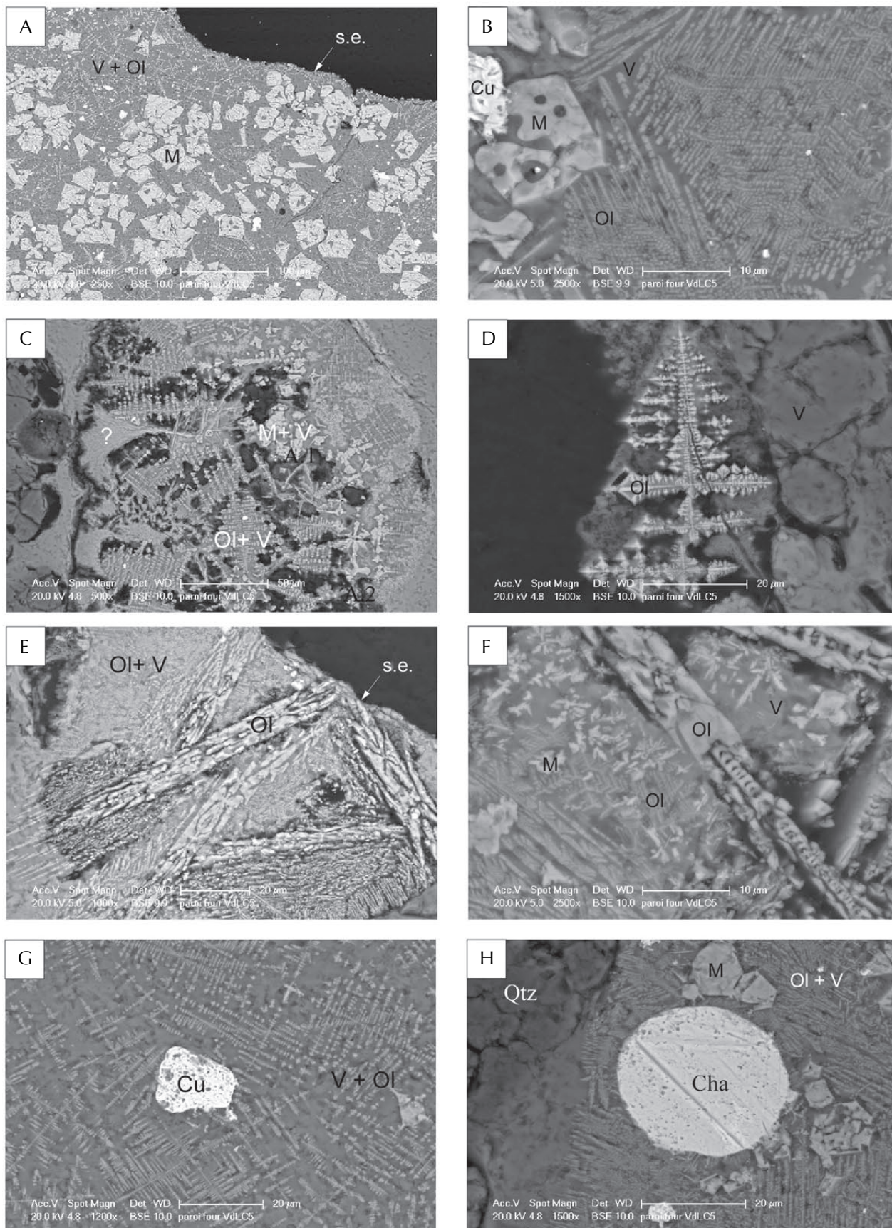
Fig. 13. Micrographies électroniques en électrons retroréfléchies du fragment de roche montrant les différents assemblages minéralogiques rencontrés dans la zone de scorie (notés A.n). Les abréviations utilisées dans les planches sont les suivantes: A.n assemblage minéralogique n / Cha chalcocite / Cu particule de cuivre / M magnétite / OI olivine / Phy phyllosilicates / Qtz quartz / R résine / S scorie / s.e. surface externe / Spl spinelle / V verre.
