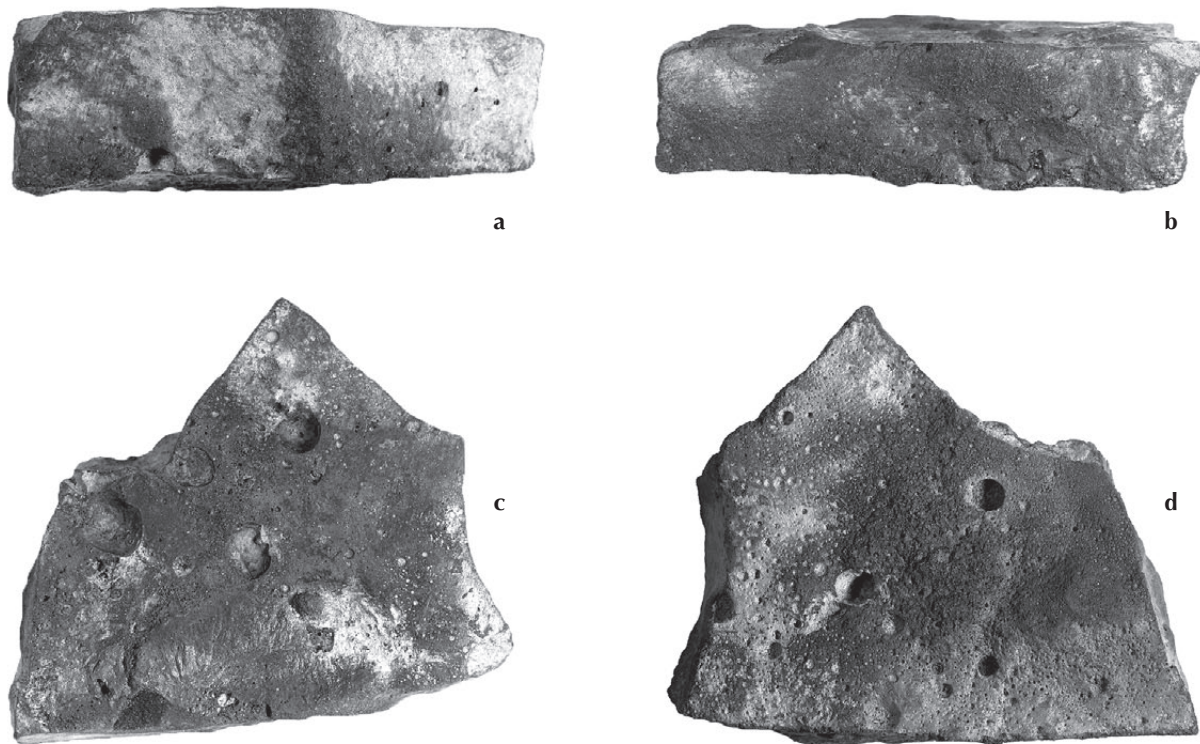
Fig. 6. Vues générales du plus gros fragment de scorie retrouvé sur le site (n° 67773), dont la morphologie est bien représentative du corpus de scories mises au jour : a) tranche (zone de fracture, épaisseur 1,6 cm), b) tranche (bord, env. 6,5 cm de longueur), c) surface supérieure montrant les zones vitrifiées noires, d) surface inférieure (photos C2RMF/D. Bagault).
