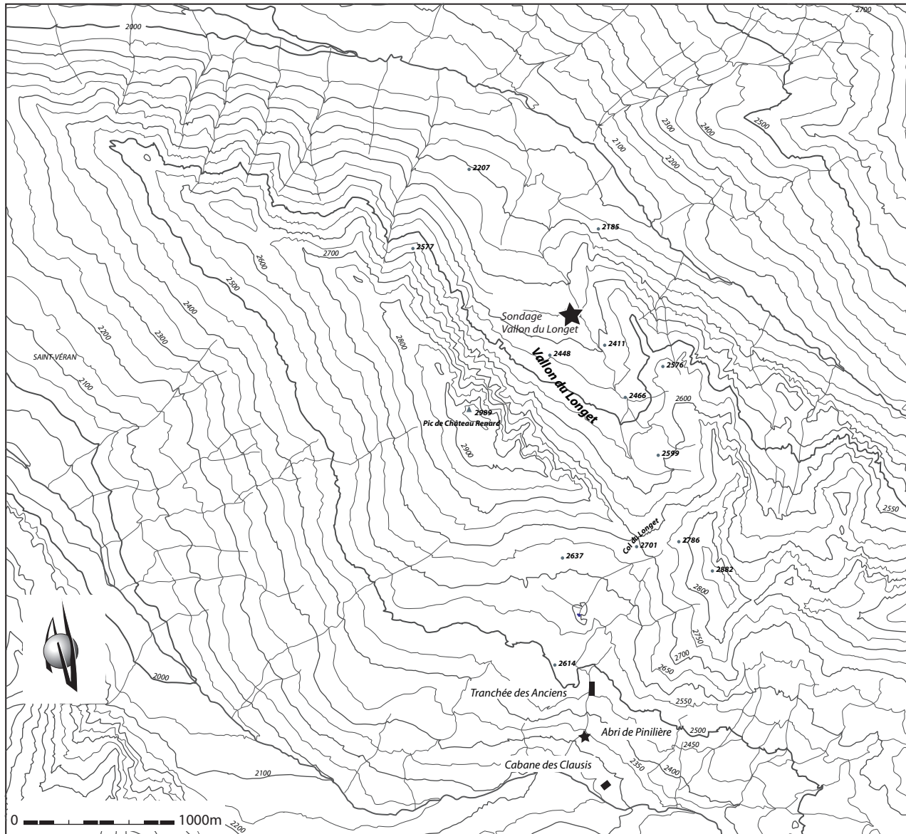
Fig. 1. Carte des principaux sites liés à l'exploitation des ressources cuprifères durant l'âge du Bronze dans la zone de Saint-Véran et de Molines-en-Queyras (Hautes-Alpes) (DAO A. Burens).
