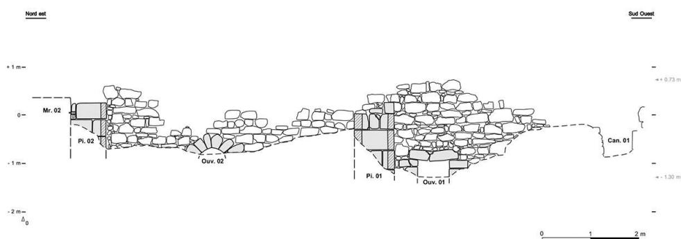
Fig. 2 – Élévation du mur gouttereau nord de l'église du prieuré de Montaigut.
