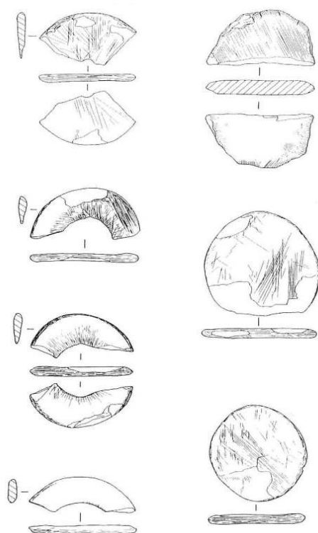
Fig. 1 – Disques, anneaux et bracelets en schiste
