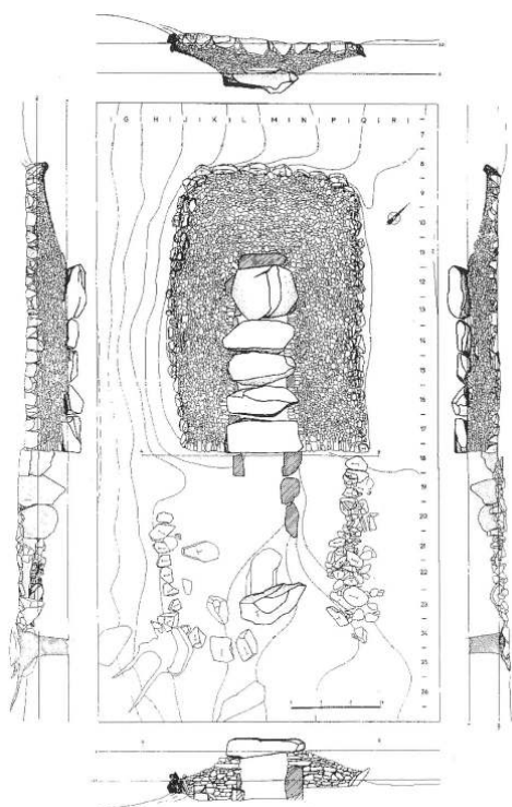
Fig. 2 – État du monument après restauration : plan et élévations des façades
