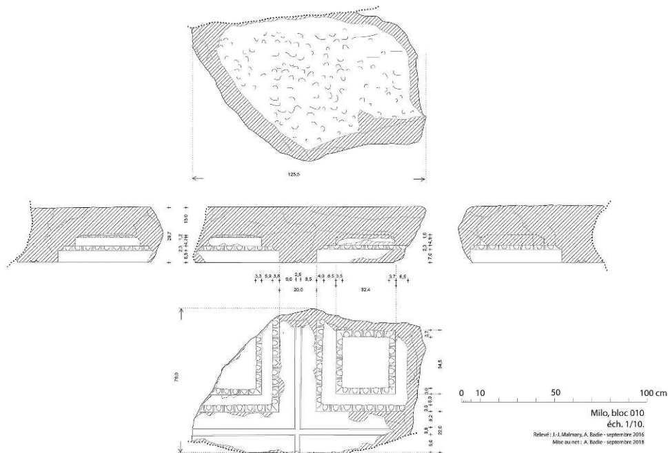
Fig. 1. La plaque de caissons 10 : relevé au 1/10 reproduit au 1/20.
