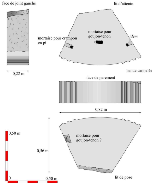
Fig. 1 – Assise de monoptère : relevé du bloc et essai d'interprétation de ses caractéristiques architectoniques
