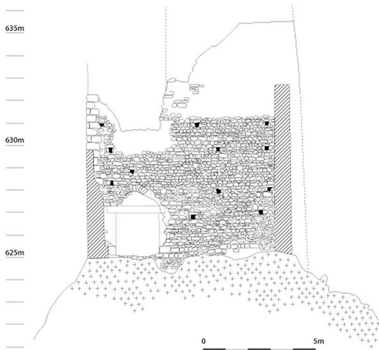
Fig. 3 – Relevé de l'élévation sud de la tour
