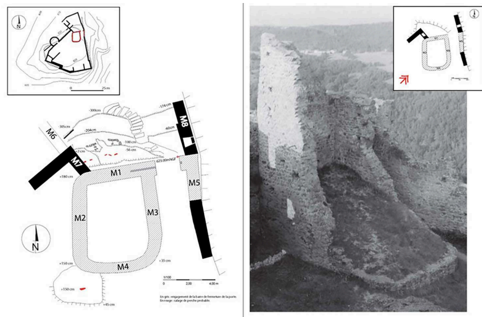
Fig. 2 – Plan et vue de la tour porche
