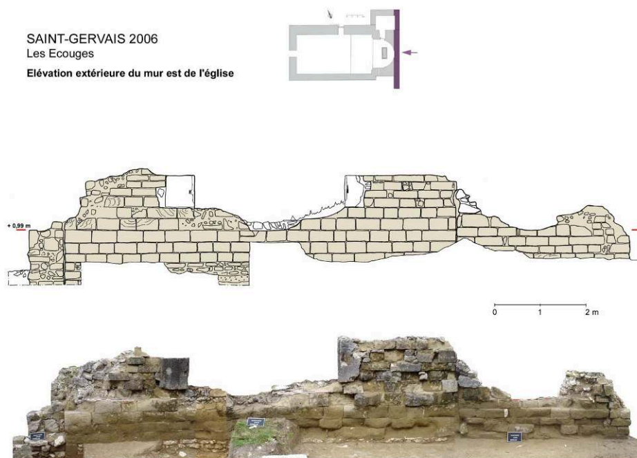
Fig. 2 – Élévation extérieure du mur est de l'église
