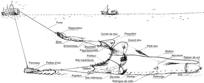
Figure 7.1. Le train de pêche (Fontaine et al. , 1979)
