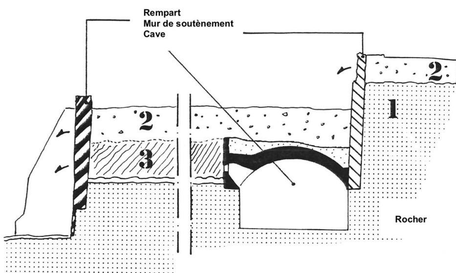
Fig. 2 – Coupe schématique
