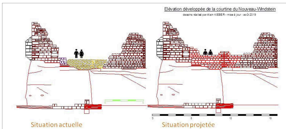
Fig. 3 – Mur nord du bastion dans sa configuration actuelle (à gauche) et dans la situation restaurée projetée (à droite)
