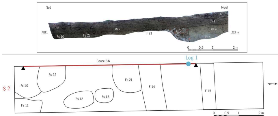
Fig. 1 – Coupe sud-nord et plan du sondage 2 : fosses antiques
