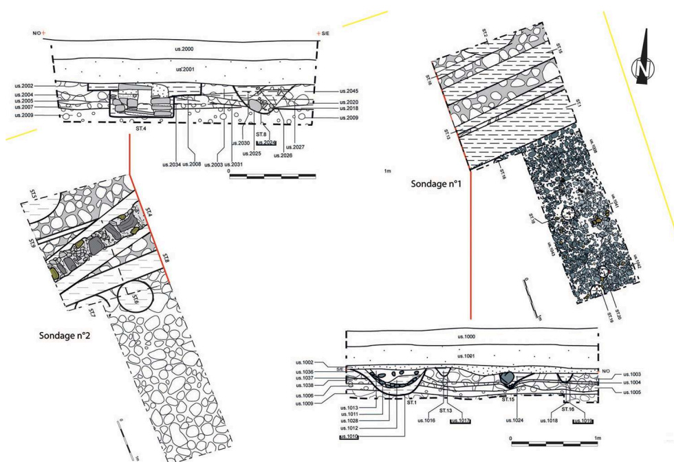
Fig. 2 – Plan de l'opération et des coupes
