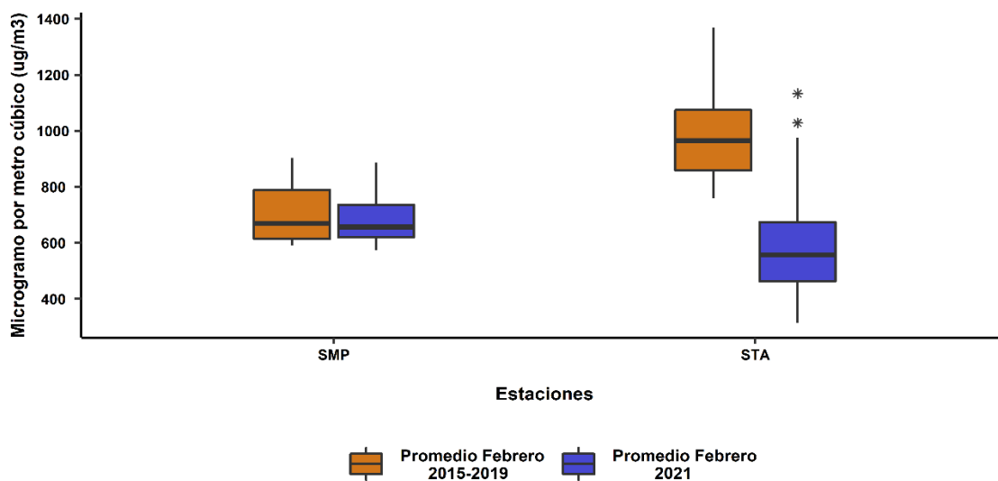
Figura N° 21. Comparativo entre las concentraciones históricas y las registradas durante el estado de emergencia para el CO
