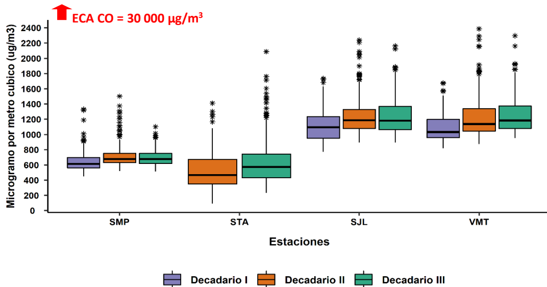
Figura N° 20. Variación horaria del CO ( \mu\text{g}/\text{m}^3 ) en el AMLC.
