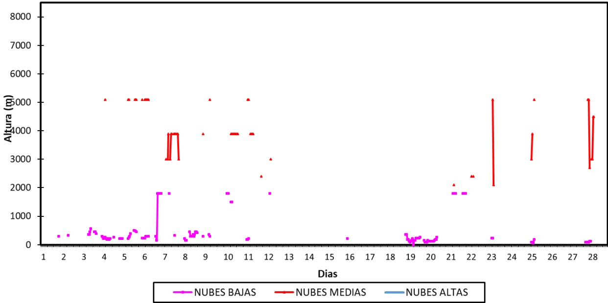
Figura N° 05. Altura de la base de nube (m) registrada en la estación Aeropuerto Internacional Jorge Chávez (JCH).
