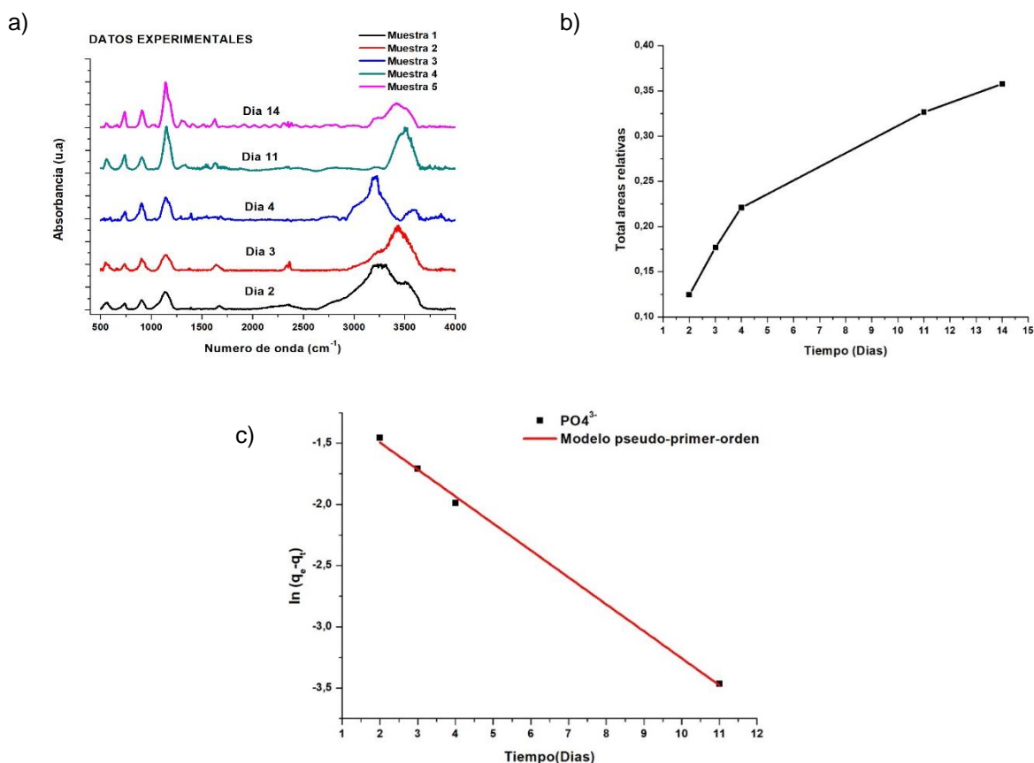
Figura 3. a) Evolución de los espectros infrarrojos de las muestras en los diferentes días de inmersión en SBF. Las bandas principales se encuentran en un rango alrededor de los 500 a 1400 cm^{-1} , alusivas a bandas de fosfato; b) gráfico del incremento de las áreas totales relativas de las bandas de fosfato; c) cinética de adsorción de PO_4^{3-} en el biovidrio durante el proceso de biomineralización representado por medio de un modelo cinético de pseudo- primer-orden.
