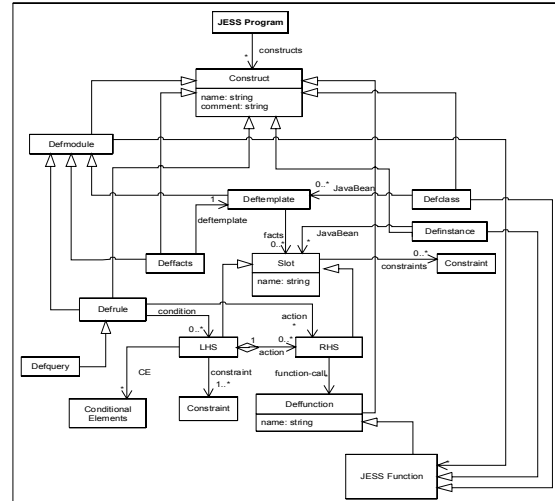
Fig. 5. Jess Meta-model
