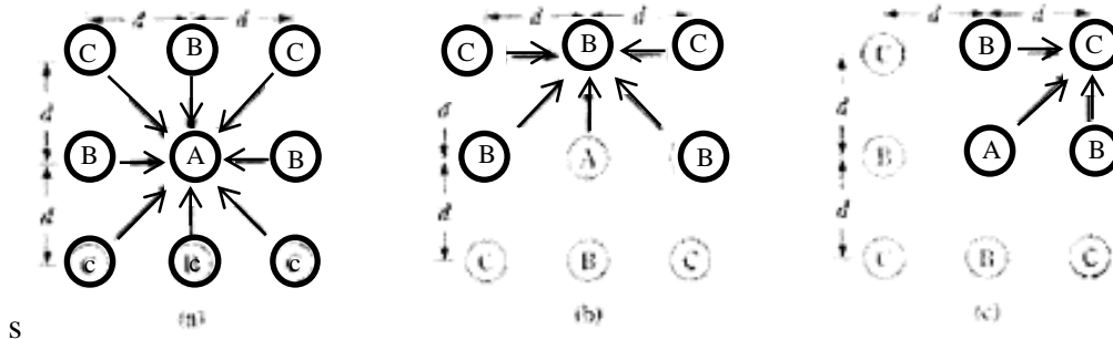
Hình 1. Hệ số nhóm cọc gần đúng theo Feld (1943)
