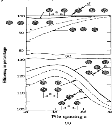
Hình 5. Các nghiên cứu trước đây của Terzaghi và Peck (1967)
