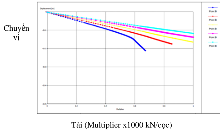
Hình 3. Các đường cong tải – chuyển vị khi khoảng cách thay đổi
