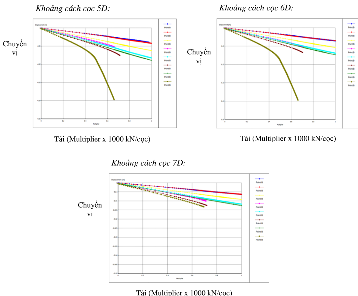
Hình 4. Các đường cong Tải – Chuyển vị khi số cọc thay đổi, với các bài toán có khoảng cách tim cọc từ 3D đến 6D
