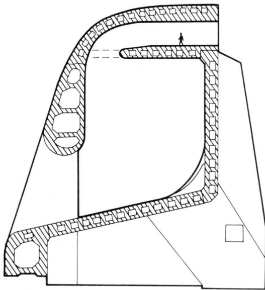
NEL Breakwater
