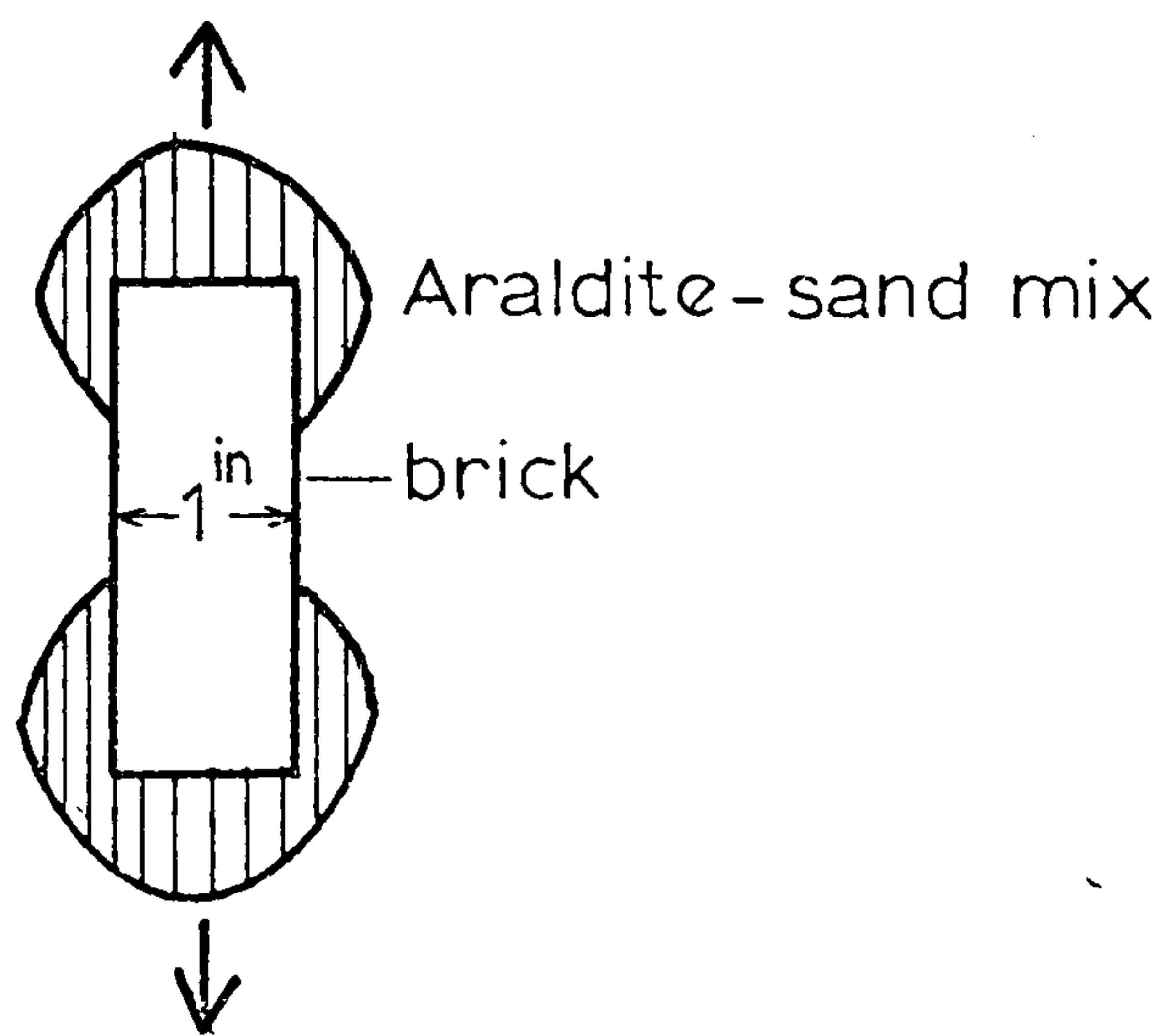
Fig.(A3) Brick tensile test
