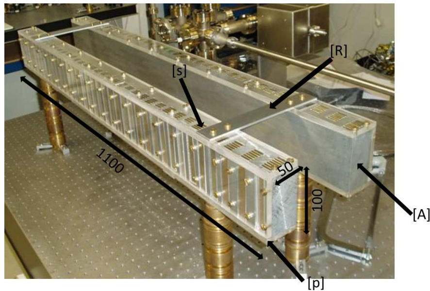
Figure 7.11: Photo de la configuration dipôle: [A] structure en aluminium, [s] sillons de profondeur variable, [p] protections en plexiglass, [R] plaques de renfort. Dimensions en mm.
