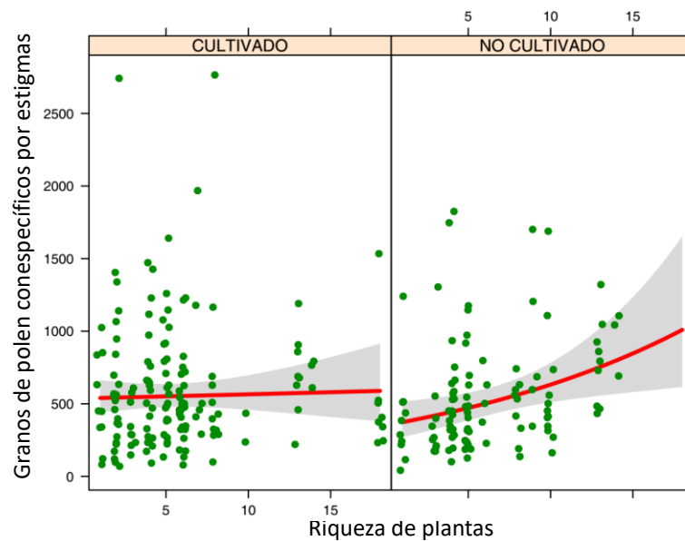
Figura 4.10 Valores residuales parciales del modelo con el número de granos de polen conespecífico por estigma en relación a la riqueza de plantas en los ELP. Izquierda: ELP adyacentes a lotes cultivados. Derecha: ELP adyacentes a lotes no cultivados. Las líneas continuas indican el ajuste del modelo entre las variables. Las líneas grises a cada lado representan el intervalo de confianza del 95%.
