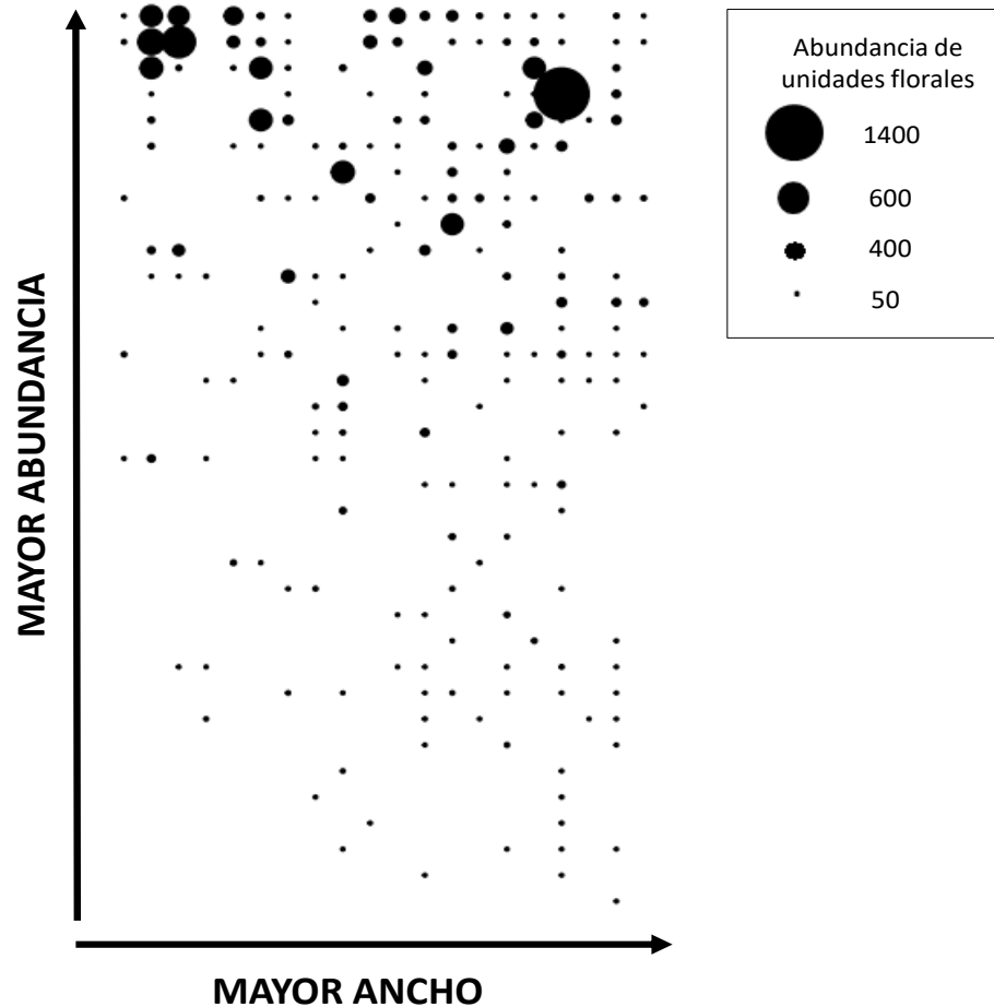
Figura 2.10. Matriz donde se muestran los 20 ELP en columnas ordenadas por el ancho, y la abundancia de flores de cada sitio en filas, donde cada punto en una misma fila es una especie. Las cuatro últimas columnas corresponden a los sitios de referencia de 40 m. El tamaño de cada punto representa el logaritmo de la abundancia de flores de las especies en ese sitio. En este gráfico no se muestran las especies con abundancias menores a 50 unidades florales.
