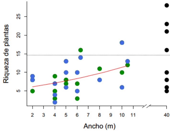
Figura 2.6. Riqueza de plantas en relación al ancho de los ELP en los sitios seleccionados. Los puntos verdes y azules corresponden a los sitios muestreados del gradiente de anchos (2-11 m) en la primera y segunda temporada de muestreo, respectivamente. Los puntos negros son los sitios de referencia (40 m). La línea punteada indica el promedio de la riqueza de plantas de estos últimos sitios, y la línea roja indica el ajuste del modelo entre las variables.
