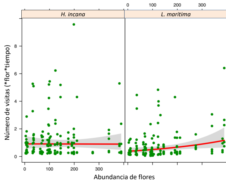
Figura 4.5 Valores residuales parciales del modelo con el número de visitantes florales (por flor y por tiempo) en los jardines de H. incana (izquierda) y L. maritima (derecha) en relación a la abundancia de unidades florales. Las líneas continuas indican el ajuste del modelo entre las variables. Las líneas grises a cada lado representan el intervalo de confianza del 95%.
