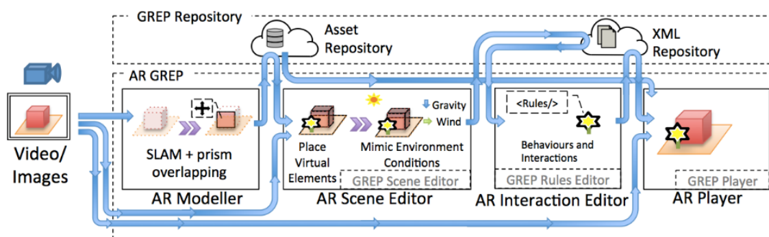
FIGURA 5.16 ARQUITECTURA DE SISTEMA AR GREP EDITOR COMPLETA [109]
