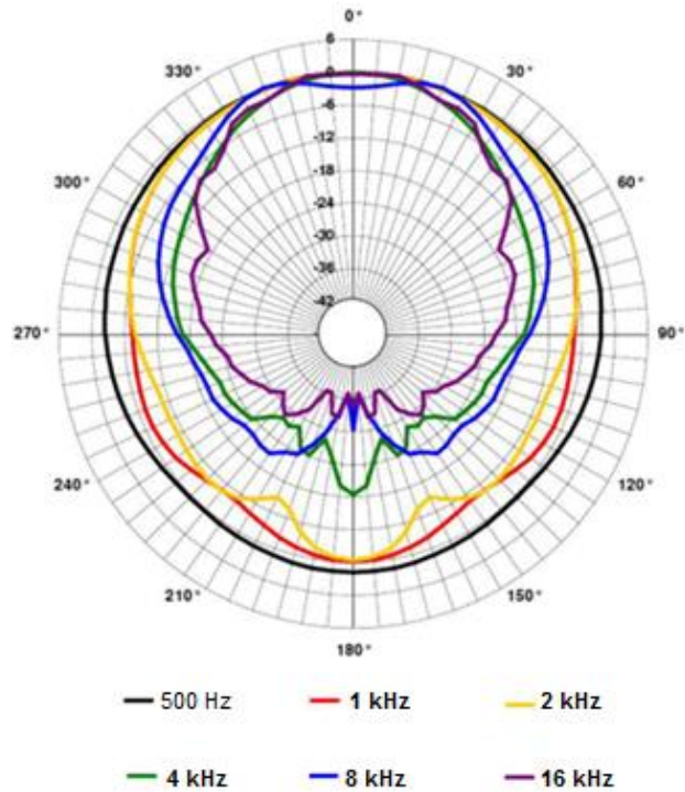
Fig. 11: Directividad de un parlante convencional.
