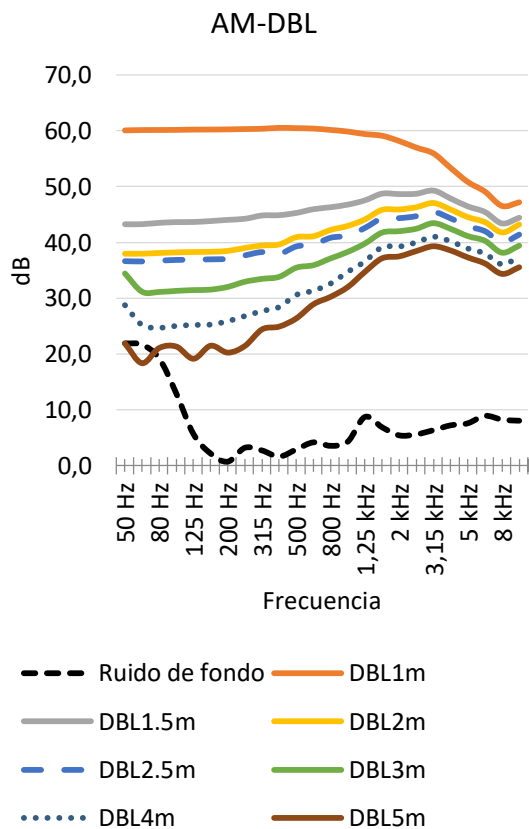
Fig. 7: Nivel de presión sonora según distancia de la modulación DBL
