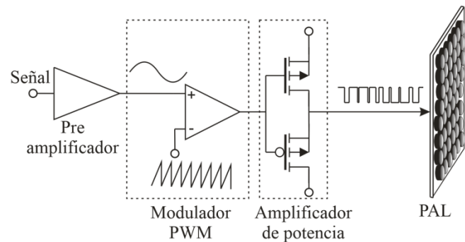
Fig. 4: Diagrama en bloques del circuito excitador PWM del PAL
