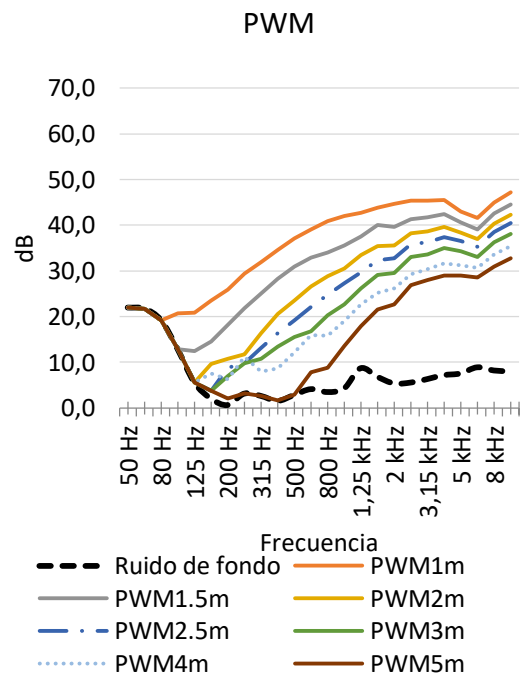
Fig. 8: Nivel de presión sonora según distancia de la modulación PWM
