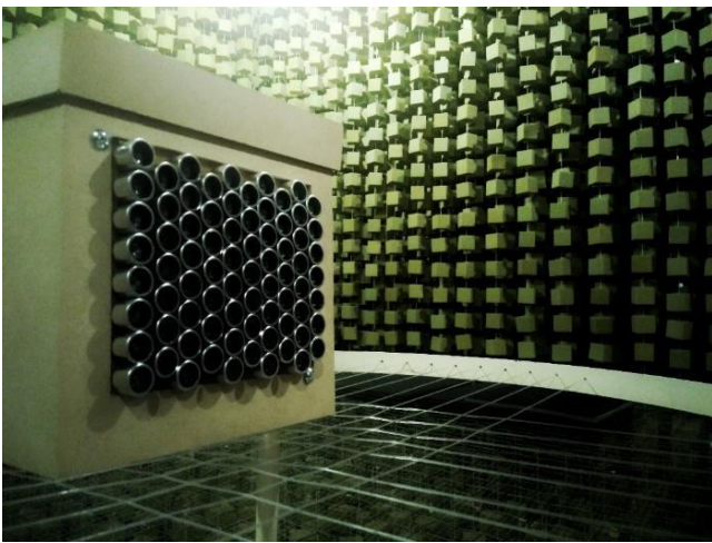
Fig. 5: PAL situado en la cámara anecoica del LAL-CIC
