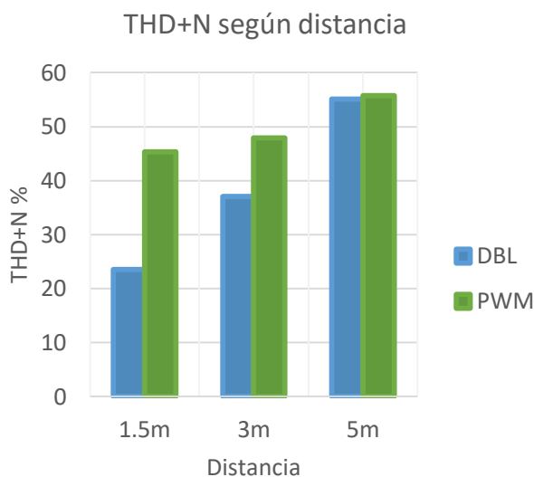
Fig. 12: THD+N de las distintas modulaciones según distancia
