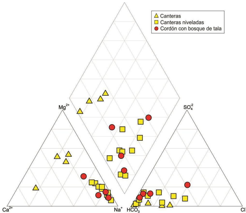
Figura 3. Diagrama Piper
