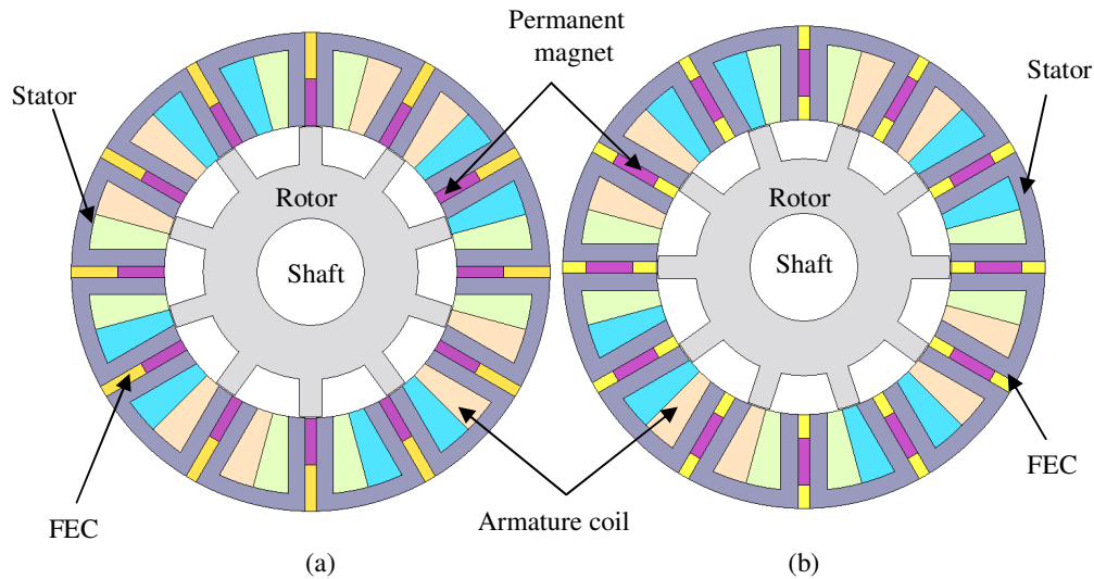
Fig. 1. 12S-10P HEFSM
