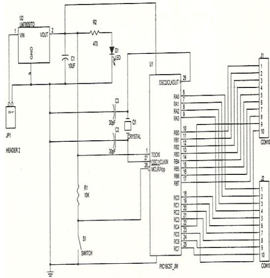
Fig. 8. Connection to/from PIC
