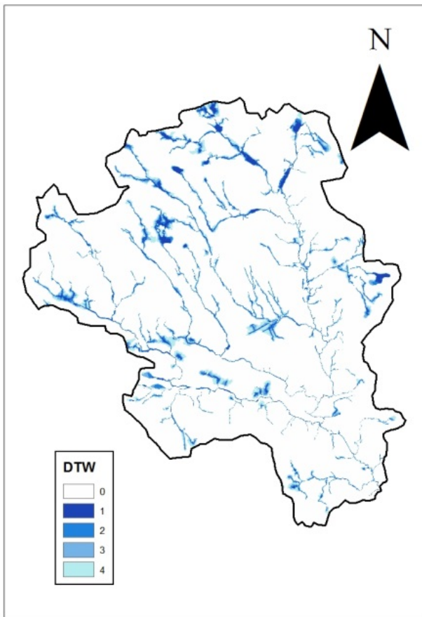
Figur 2. Figuren visar den resulterande griden med ett beräknat DTW-index för varje pixel. DTW-indexet är sedan indelat i 5 klasser, klass 0 DTW > 1 m, klass 1 DTW ≤ 0,1 m, klass 2 DTW 0,1- 0,25 m, klass 3 DTW 0,25-0,5 m och klass 4 DTW 0,5- 1 m.
